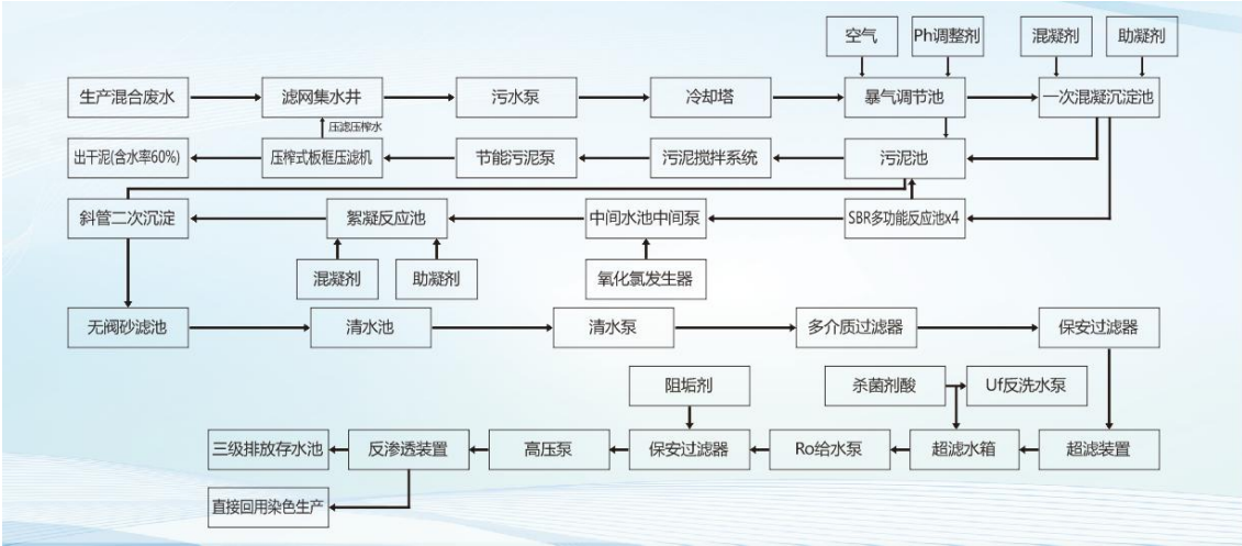
图 2-2 南厂区污水处理工艺流程图
